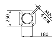
Присоединительный фланец
